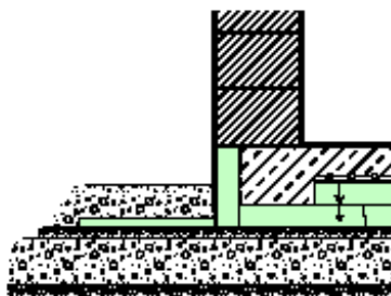
Thermobodenplatte
