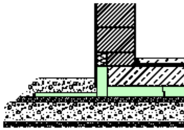
Monolithische Wandkonstruktion
