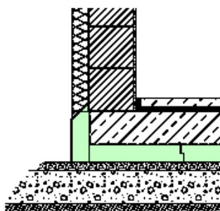
WDVS Wandkonstruktion
