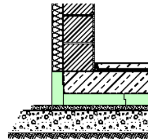
WDVS Wandkonstruktion
