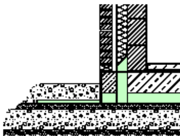
Mehrschalige Wandkonstruktion
